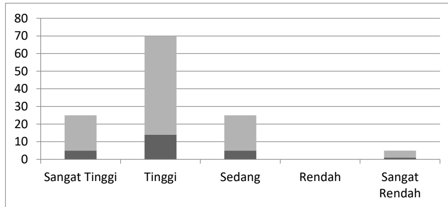
Gambar 4. Histogram Faktor Tendangan Pinalti
