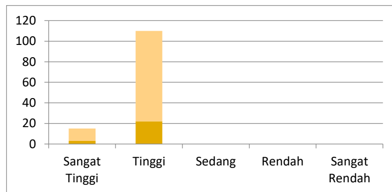
Gambar 1. Histogram Kategorisasi Data Faktor Peraturan Offside
