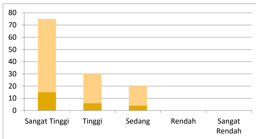
Gambar 2. Histogram Hasil Pengkategorian Data Faktor Pelanggaran Dan Kelakuan Tidak Sopan
