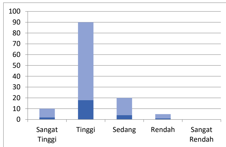
Gambar 3. Histogram Kategori Data Kategorisasi Data tingkat pemahaman wasit berlisensi faktor tendangan bebas
